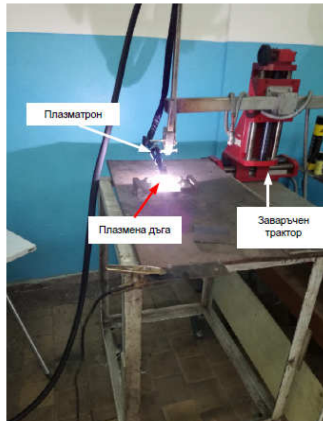
Реализиране на процеса на плазмено заваряване
