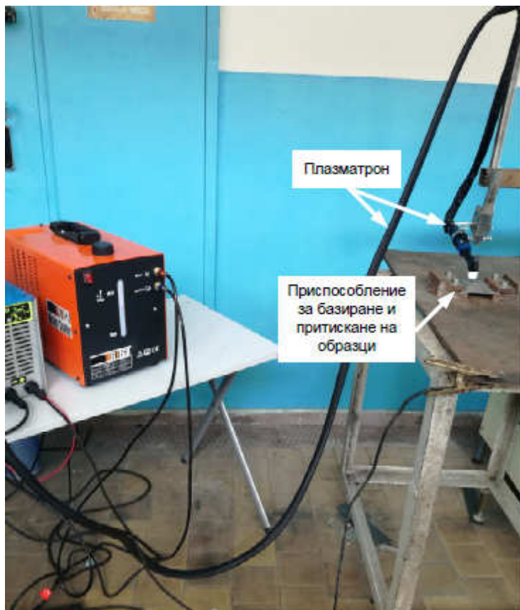
Закрепване на плазматрона и образца
