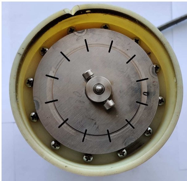
Снимка на въртящия диск на електронно-лъчев анализатор
