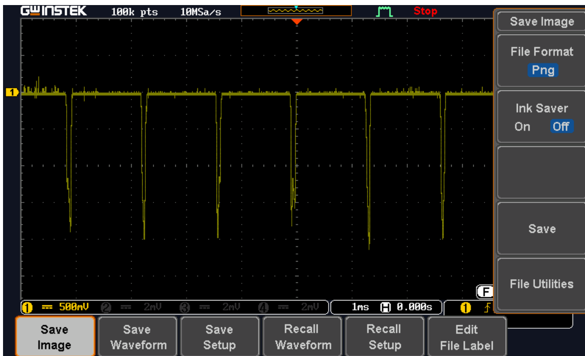
Примерен сигнал получен при ток на лъча I_{beam} = 5[mA] и ток на фокусировка I_f = 523[mA] .
